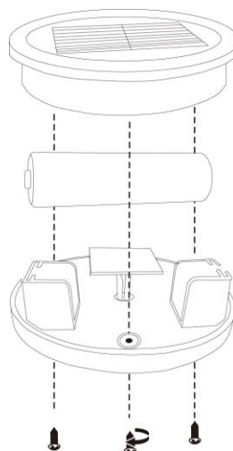
Abbildung 4: Entnahme der Batterie
