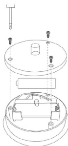
Abbildung 4: Entnahme der Batterie
