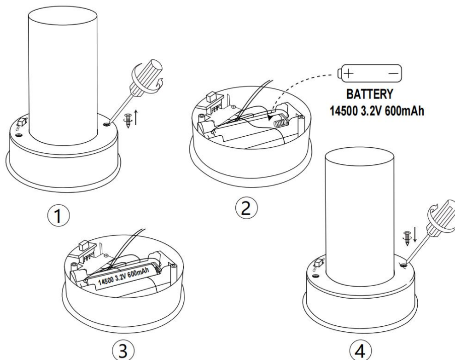
Abbildung 4: Entnahme der Batterie
